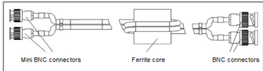
Abbildung 111: TCAS-2, TCASR-2 – CAS-Kabel C39195-A7700-B13
