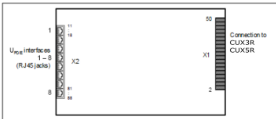
Abbildung 80: SLU8NR
