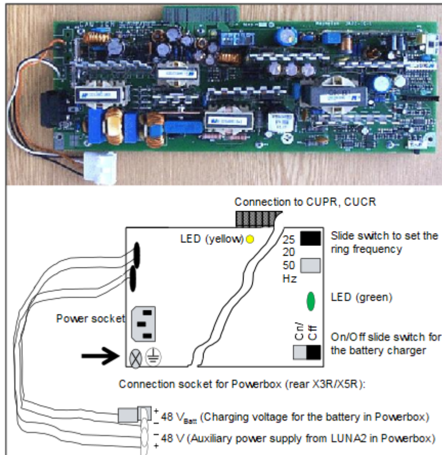
Abbildung 136: UPSC-DR
