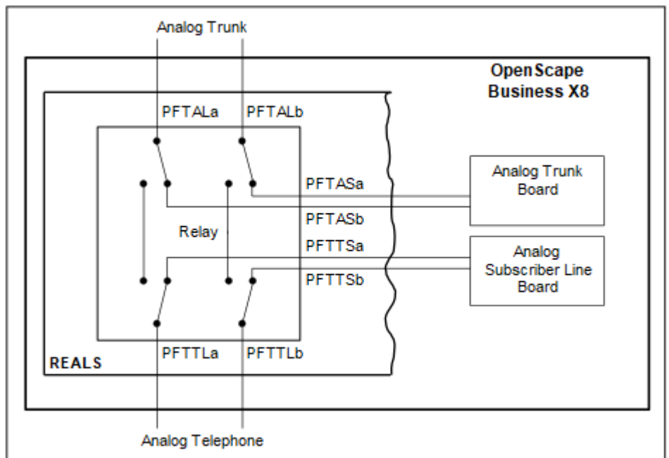
Abbildung 65: REALS – Prinzipschaltbild (Kommunikationssystem im Normalbetrieb)
