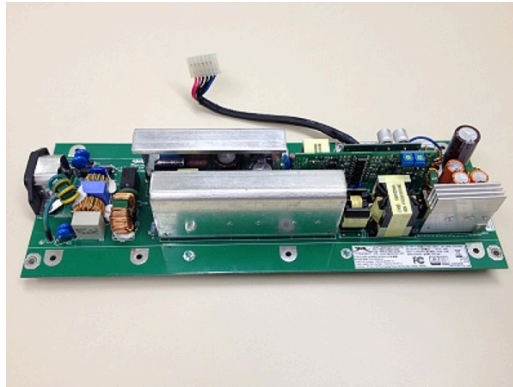
Abbildung 63: OCPSM
