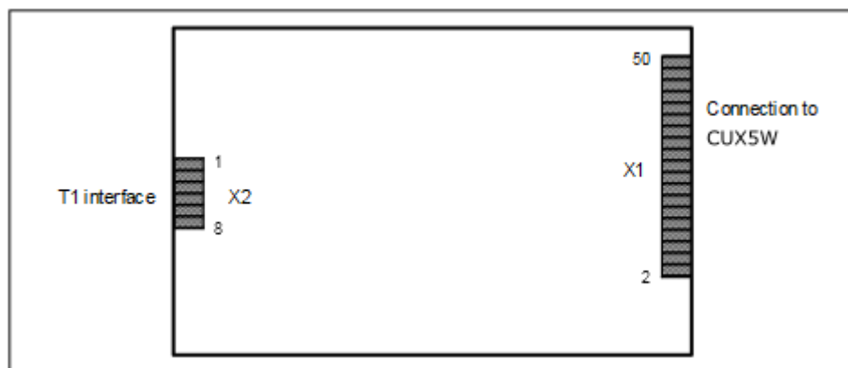
Abbildung 133: TST1
