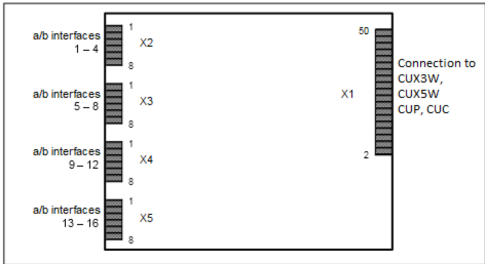
Figura 69: SLAV16
