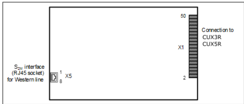
Abbildung 130: TS2RN
