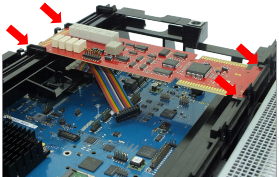
Abbildung 103: STRB einstecken
