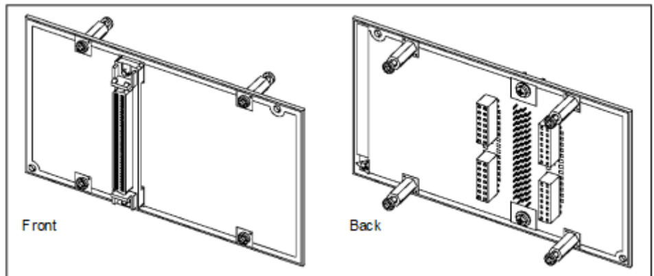
Abbildung 14: DBSAP
