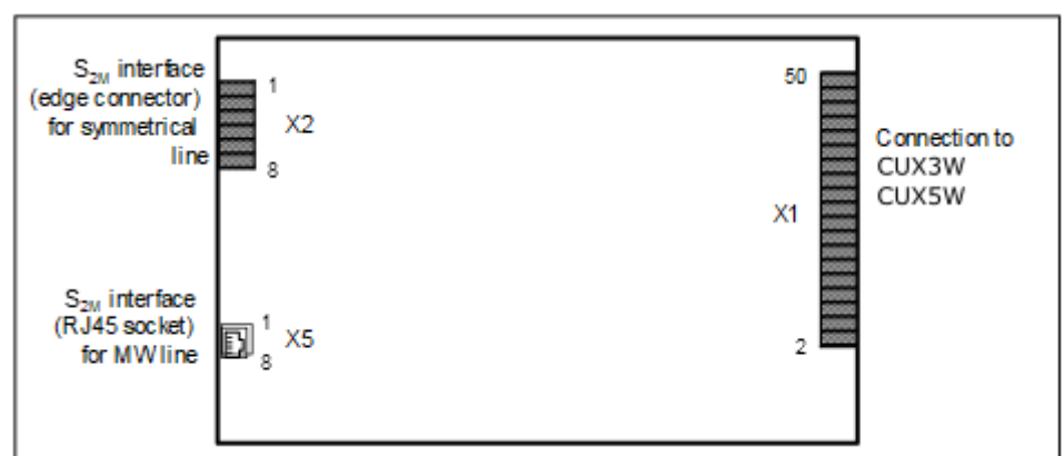
Abbildung 129: TS2N
