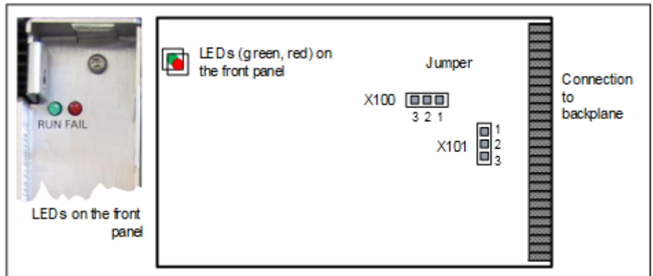
Abbildung 119: TMANI
