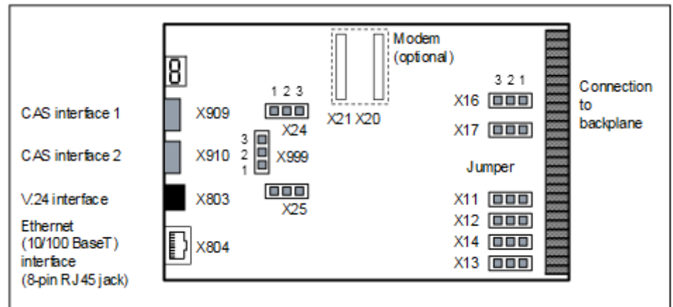
Abbildung 120: TMCAS2
