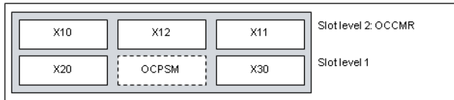
Abbildung 13: CUX3R
