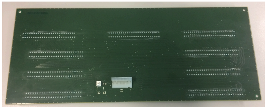
Abbildung 35: Rückwandverdrahtung CUX5W
