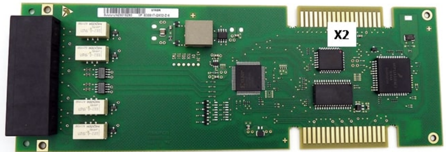
Abbildung 84: STRBR (S30817-Q932-Z ) bis zu Ausgabe 6
