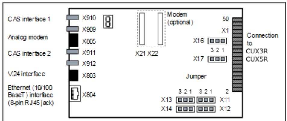
Abbildung 109: TCAS-2, TCASR-2 – Anschlüsse und Jumper
