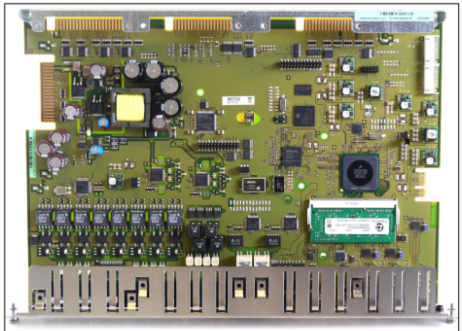
Abbildung 55: OCCMR
