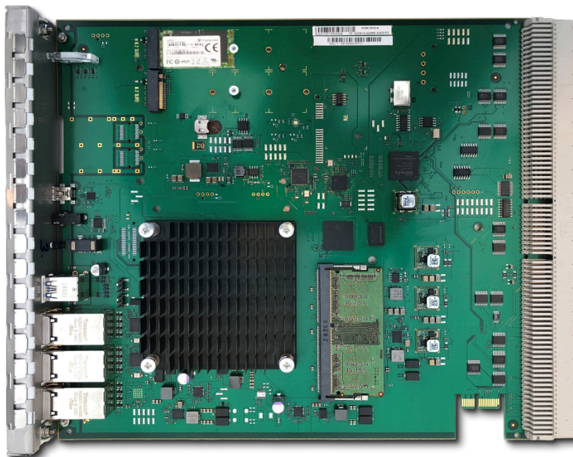
Abbildung 46: OCCLA
