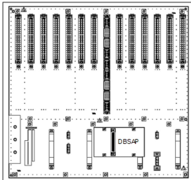
Abbildung 15: DBSAP – Montage auf der Backplane der Erweiterungsbox
