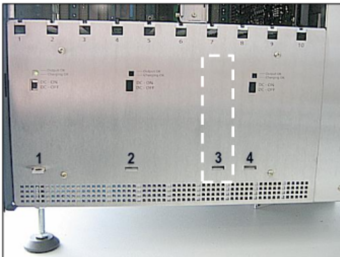
Abbildung 66: REALS – Steckplatz 3 in der Basisbox
