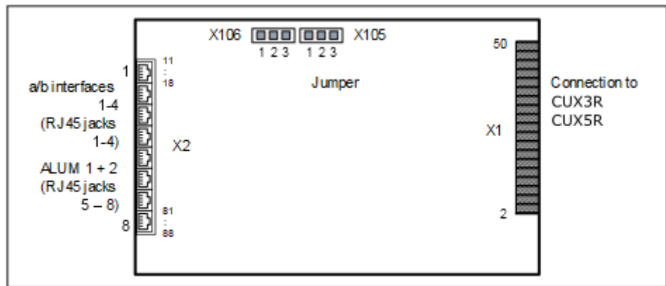
Abbildung 117: TLANI4R
