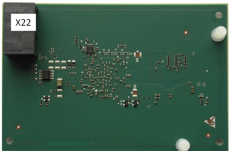
Abbildung 41: Beispiel OCCBL - Rückseite mit gesteckten Abstandsbolzen
