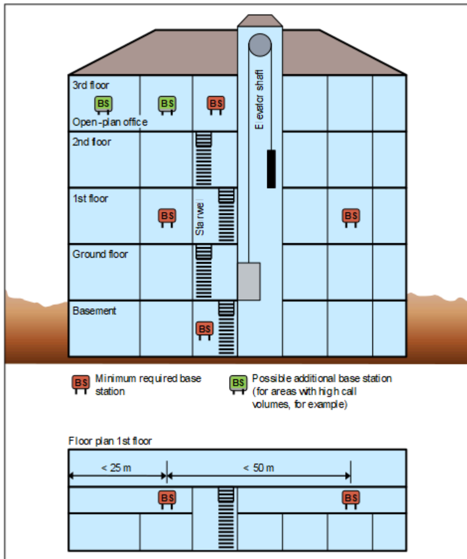
Abbildung 141: Beispiel für die Positionierung von Basisstationen in Gebäuden in Ziegel- und Leichtbauweise
