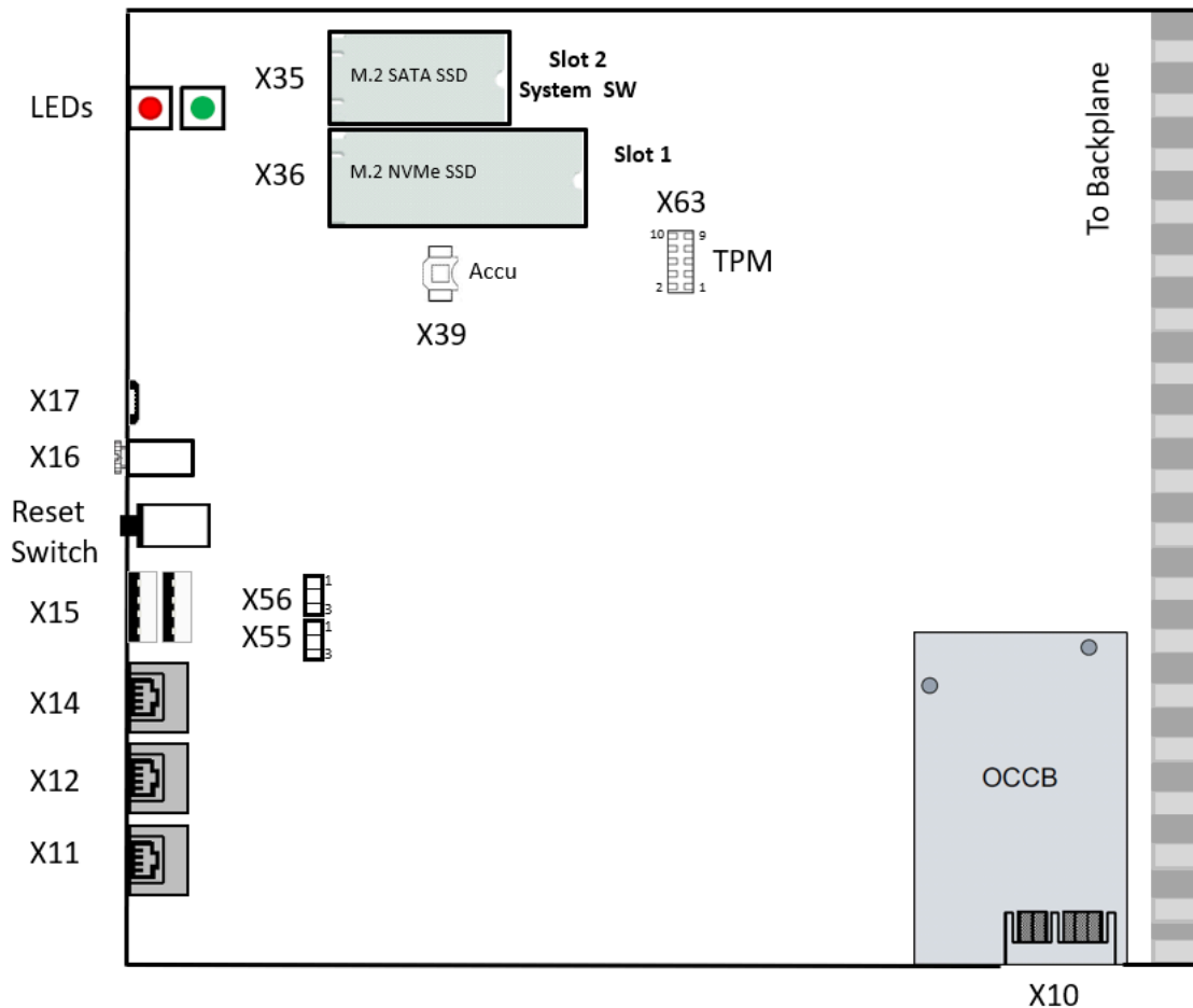
Abbildung 48: OCCLA Anschlüsse
