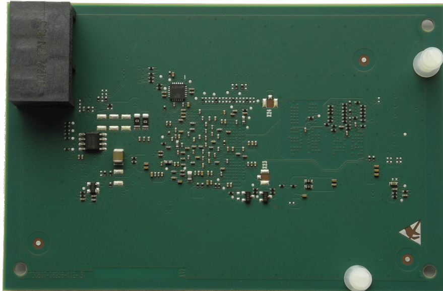
Abbildung 36: Beispiel OCCBL- Rückseite mit gesteckten Abstandsbolzen
