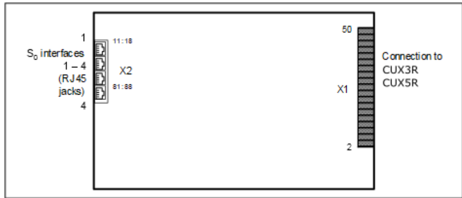
Abbildung 82: STLSX4R
