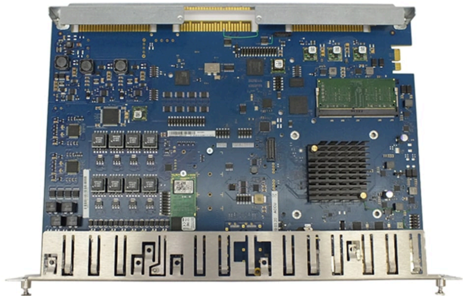
Abbildung 59: OCCMBR
