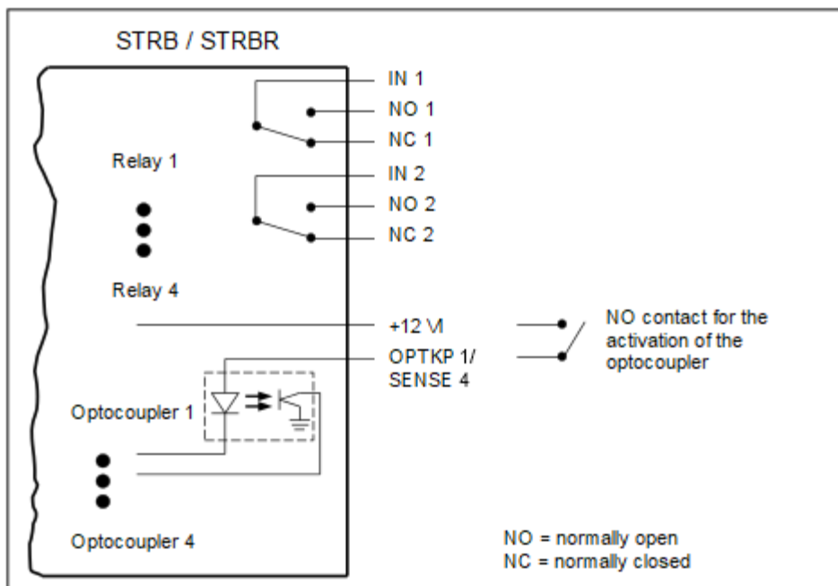
Abbildung 99: STRB, STRBR – Prinzipschaltbild
