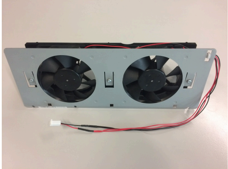
Abbildung 34: Lüfterkit (C39165-A7021-B320) für Systeme mit Rückwandverdrahtung CUX5W
