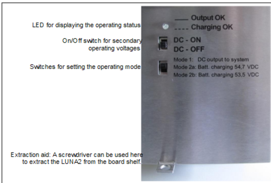
Abbildung 23: LUNA2 – Frontblende
