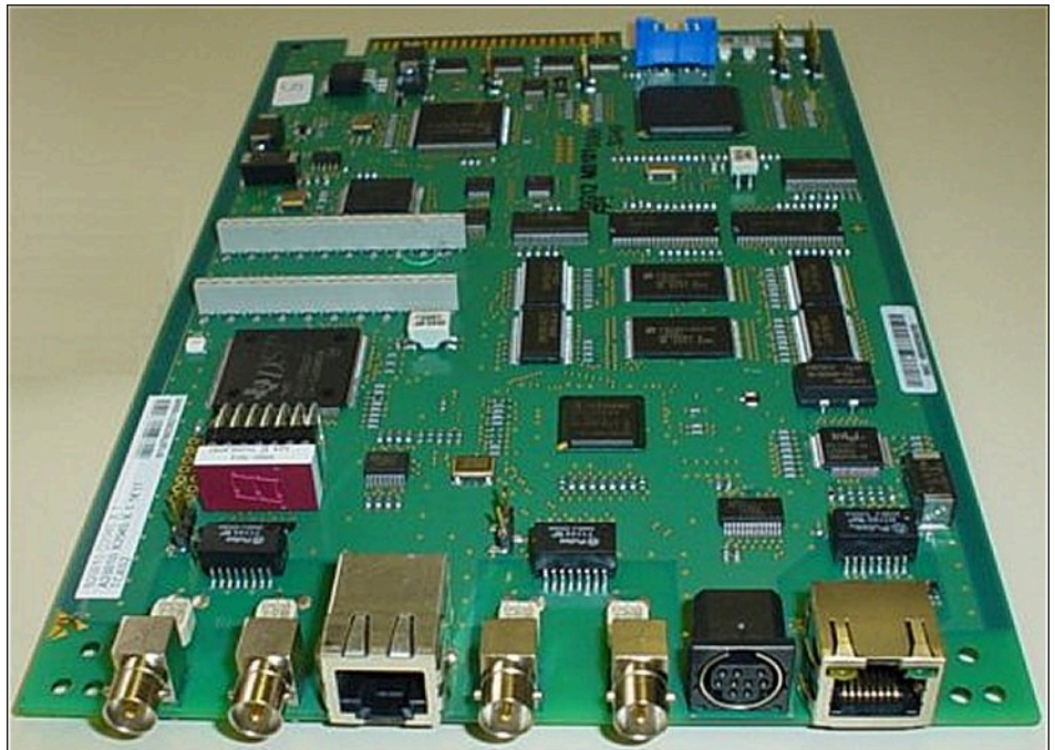
Abbildung 108: TCAS-2, TCASR-2
