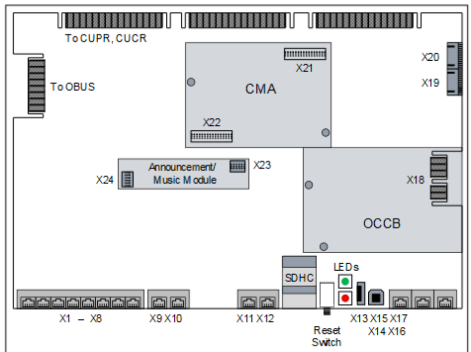
Abbildung 56: OCCMR – Anschlüsse
