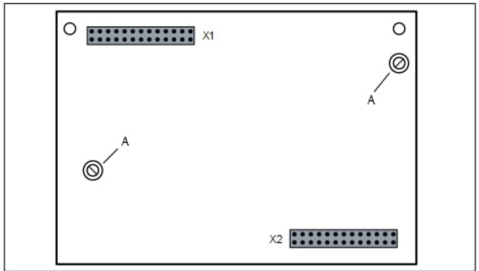
Abbildung 9: CMAe – Bestückungsseite mit gesteckten Abstandsbolzen (A)
