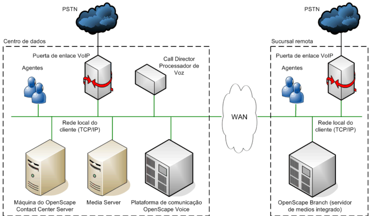
Figura 1 Configuração de rede com o OpenScape Branch
