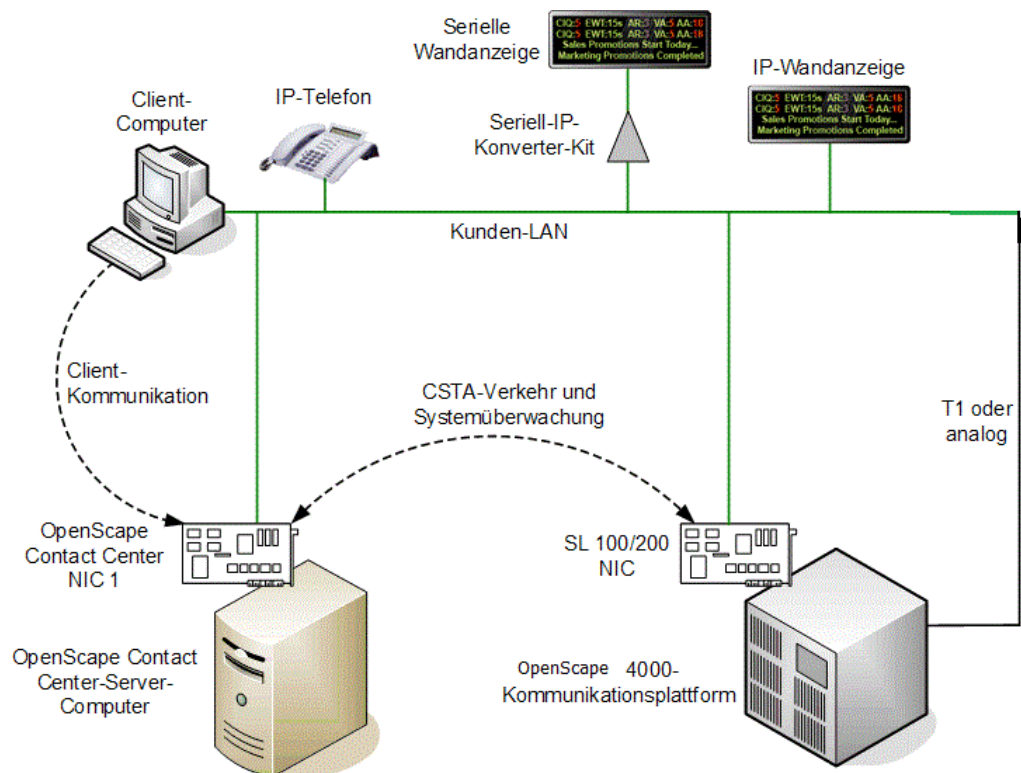
Bild 2 Netzwerkkonfiguration
