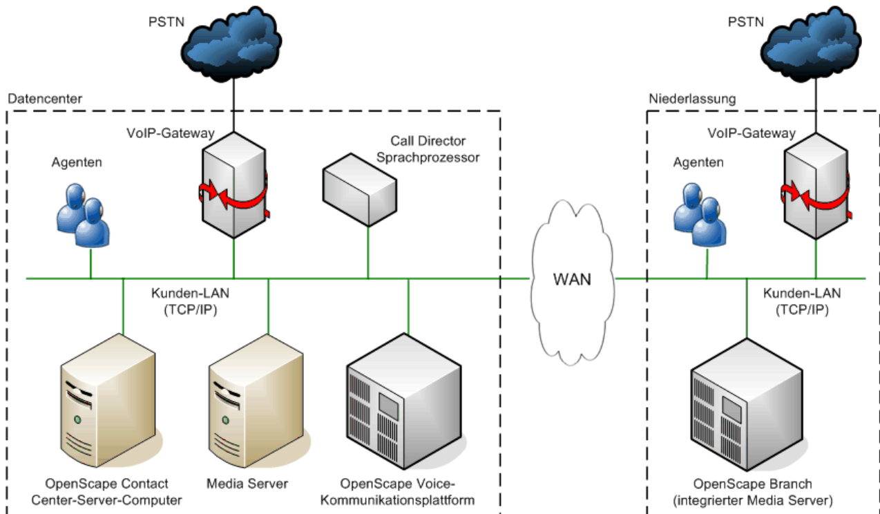
Bild 1 Netzwerkkonfiguration mit OpenScape Branch
